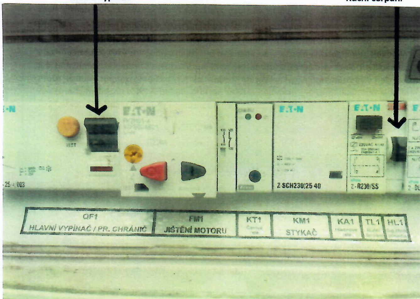
Hlavní vypínač
